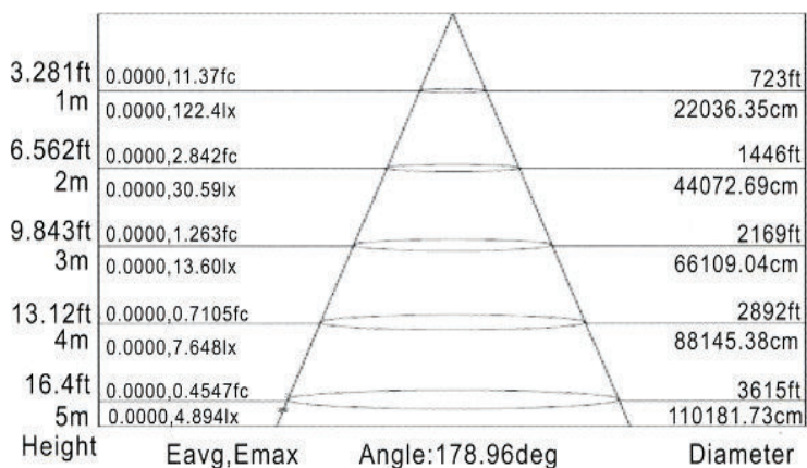
等照度曲線
