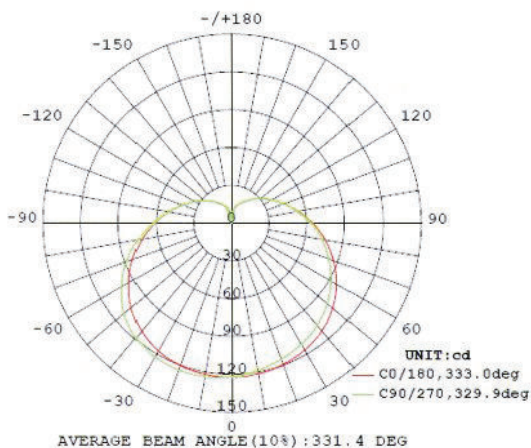
配光特性
